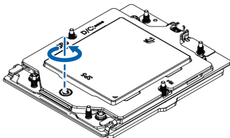
图 4-11 拧松 CPU 压板上的松不脱螺钉
