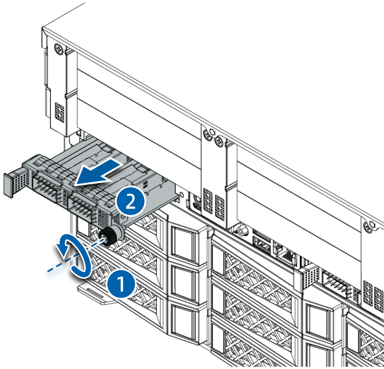
图 4-21 拆卸 OCP 3.0 网卡
