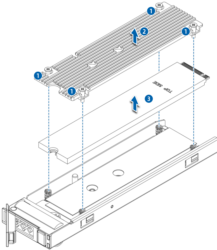
图 4-24 拆卸后置 M.2 硬盘
