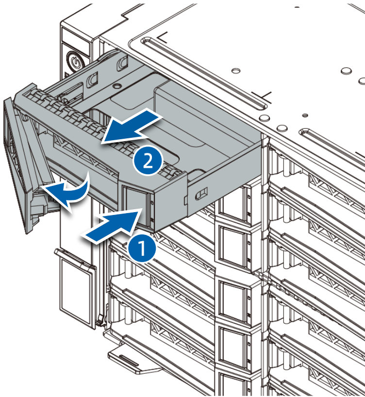
图 4-18 拆除硬盘模组
