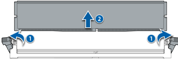
图 4-6 拆卸内存示意图
