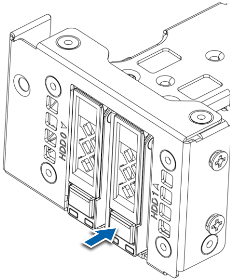
图 4-22 按压 M.2 托架按钮
