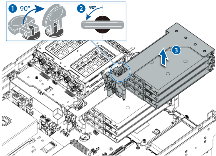
图 4-14 拆卸 PCIe 转接卡模组
