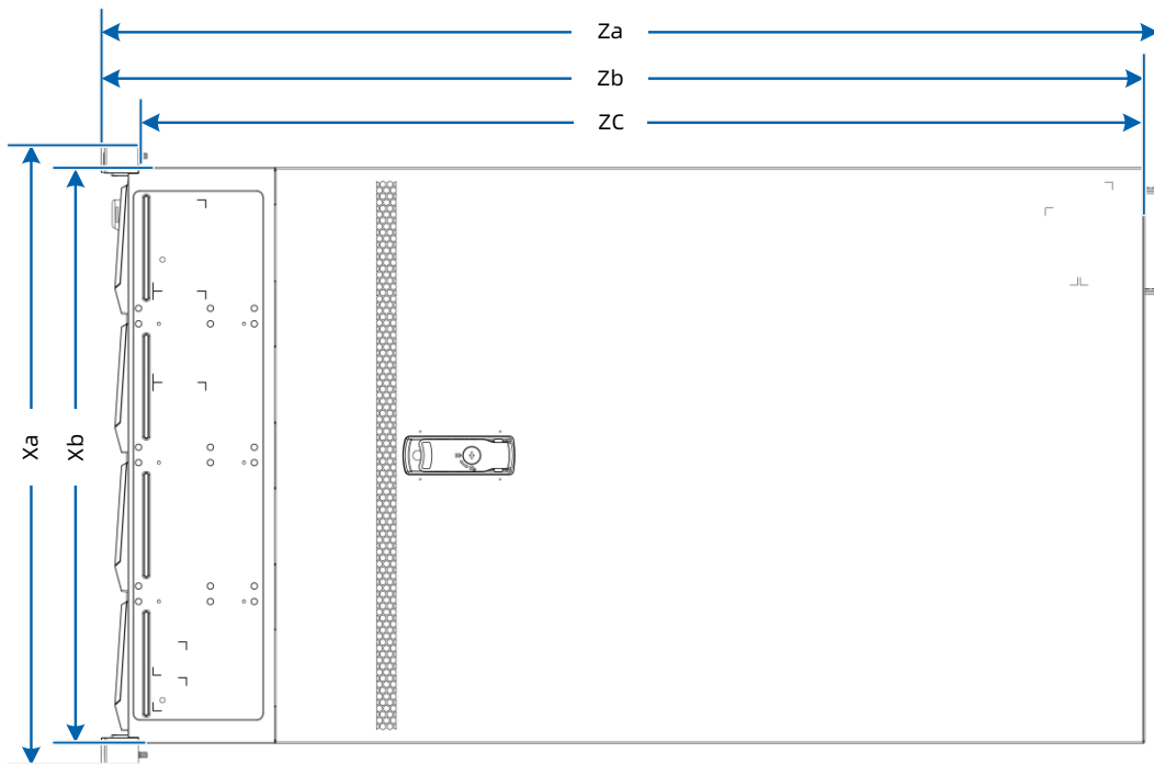
图 2-2 主机尺寸
