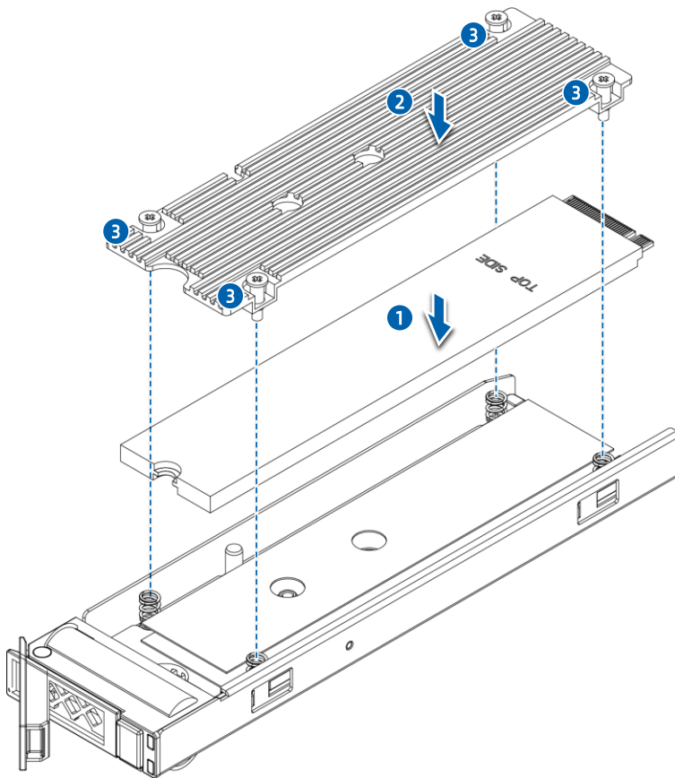
图 4-25 将 M.2 硬盘固定在托架上
