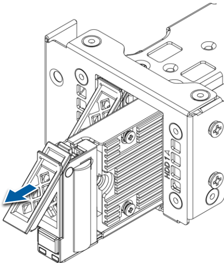
图 4-23 拉出 M.2 硬盘模组
