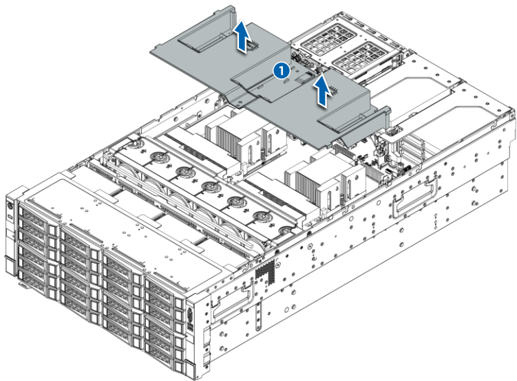
图 4-4 拆卸导风罩
