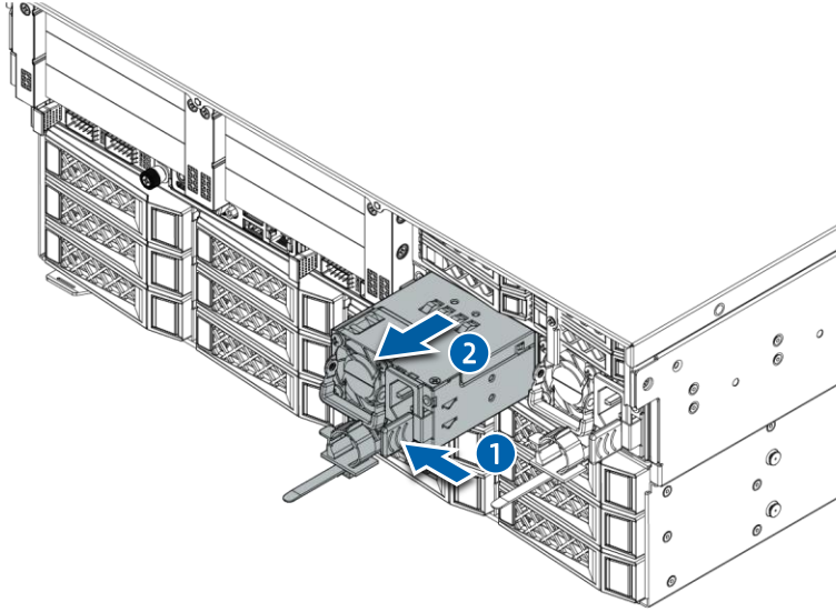
图 4-20 拆卸电源
