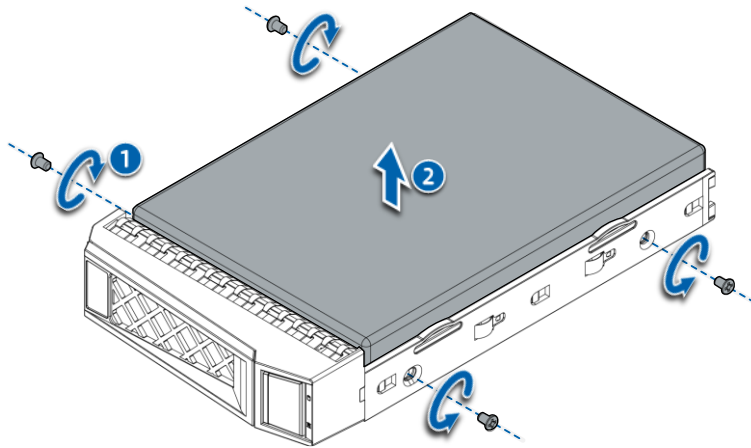
图 4-17 拆除硬盘
