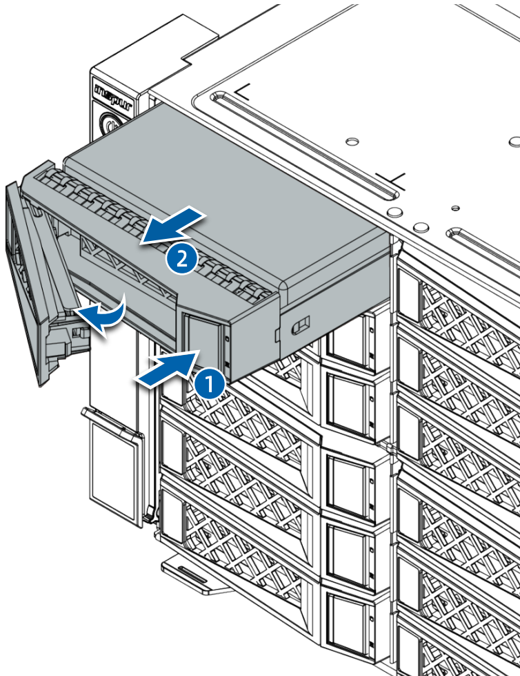
图 4-16 拆除硬盘模组
