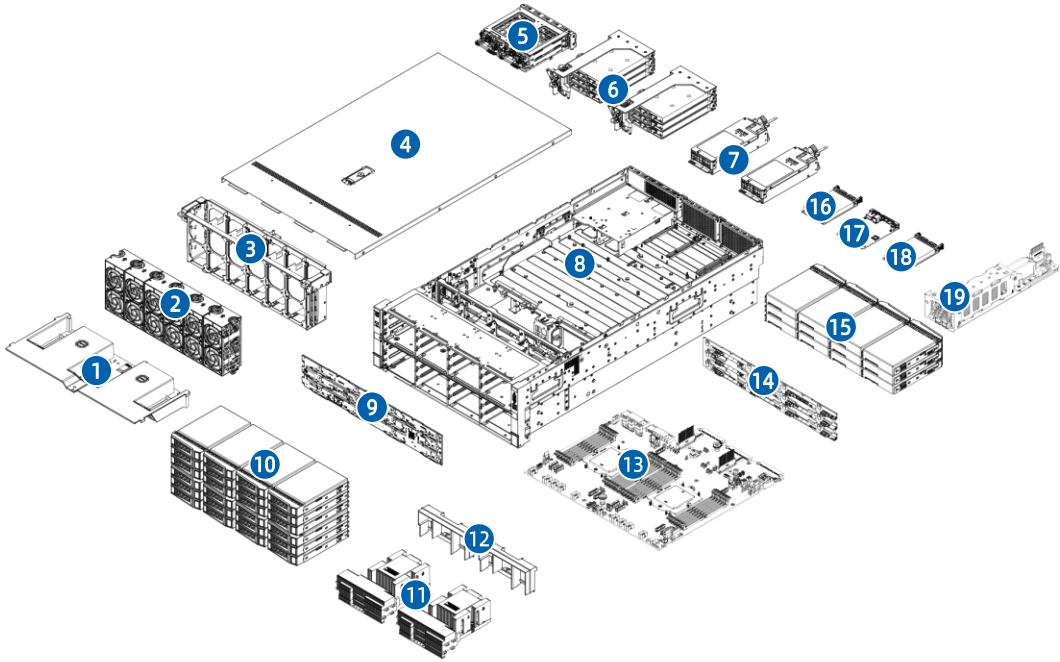
图 3-7 物理结构图
