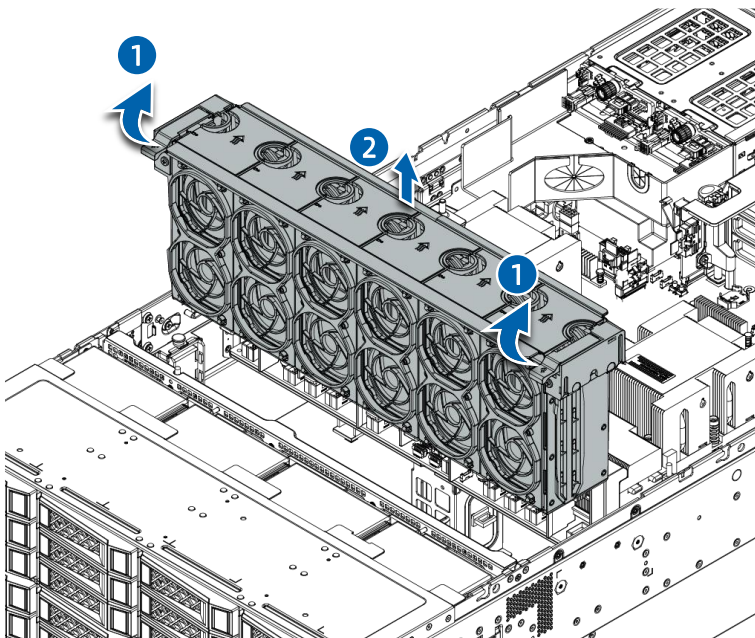
图 4-7 拆卸其它组件
