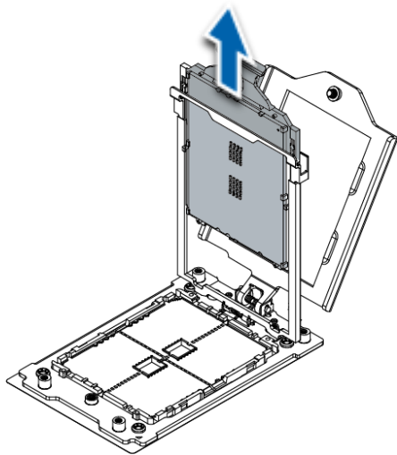
图 4-13 拆卸 CPU 套件
