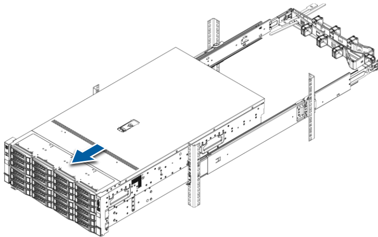
图 4-1 将服务器拉出机架
