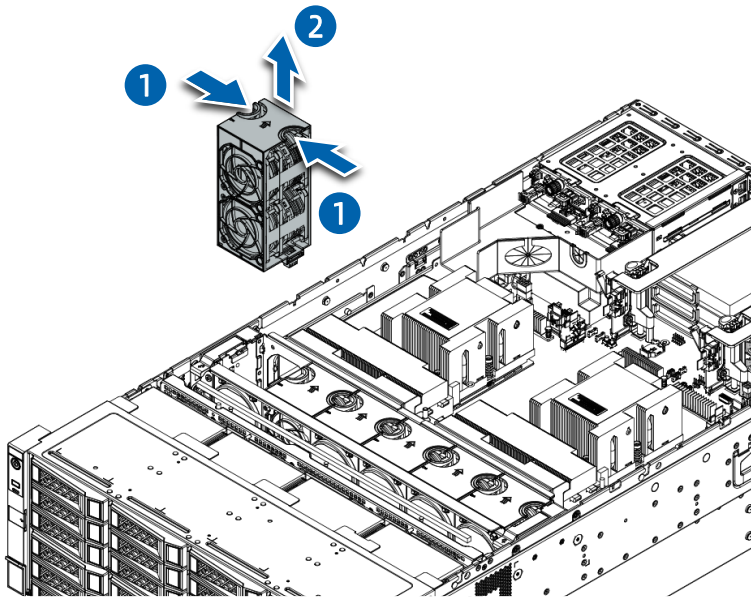
图 4-5 拆卸风扇模组
