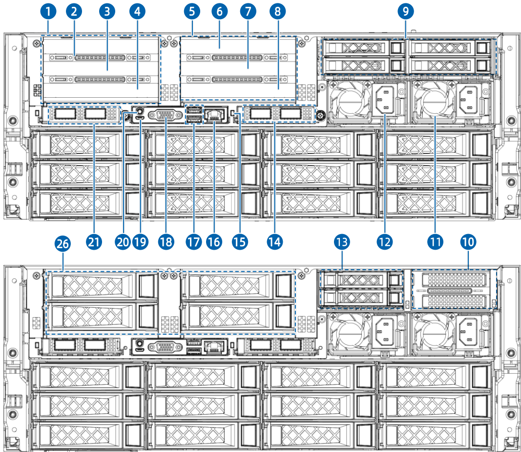
图 3-2 后面板
