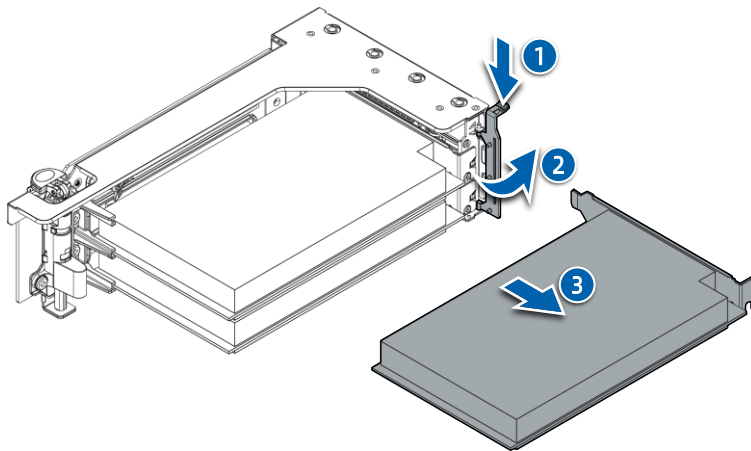
图 4-15 拔出 PCIe 扩展卡
