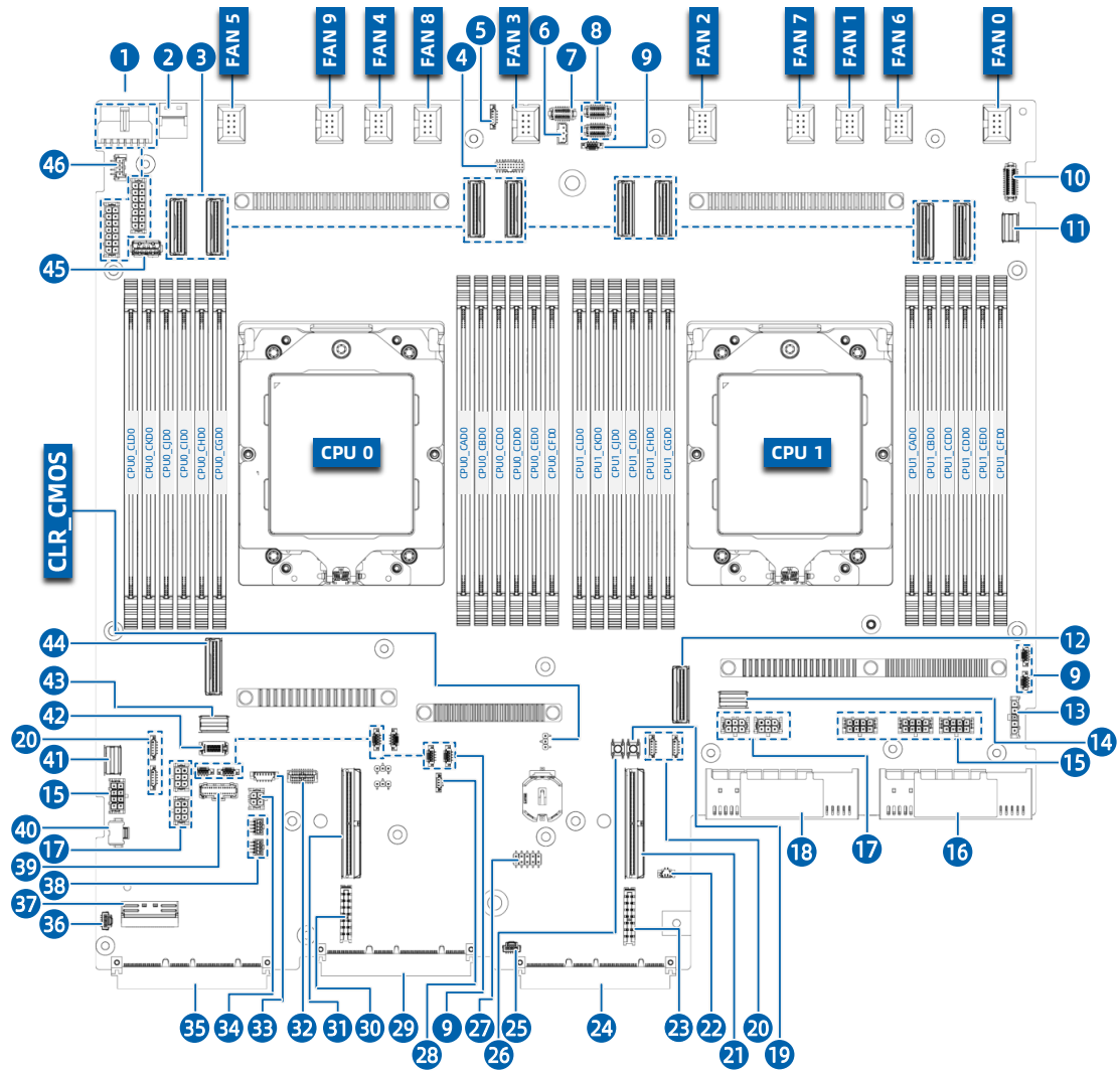
图 3-6 主板布局
