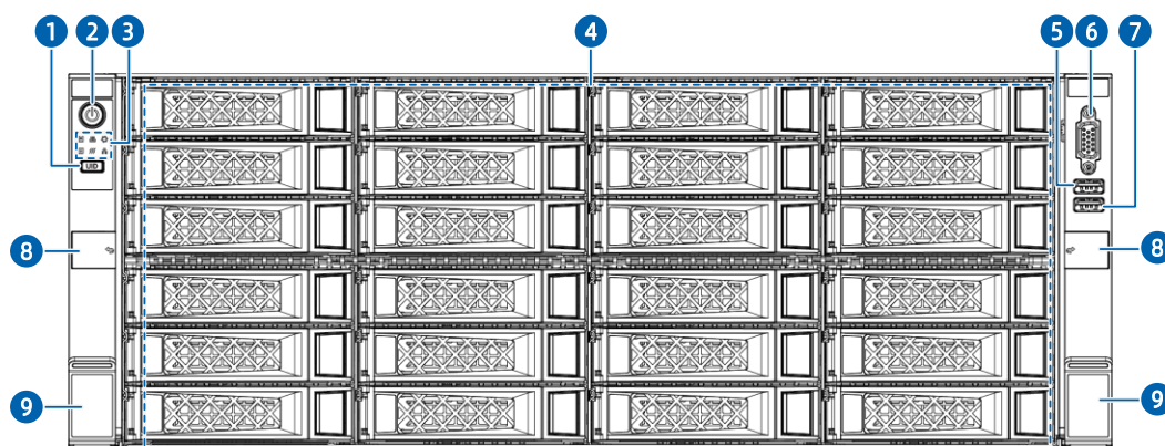
图 3-1 24 × 3.5 英寸硬盘配置前面板
