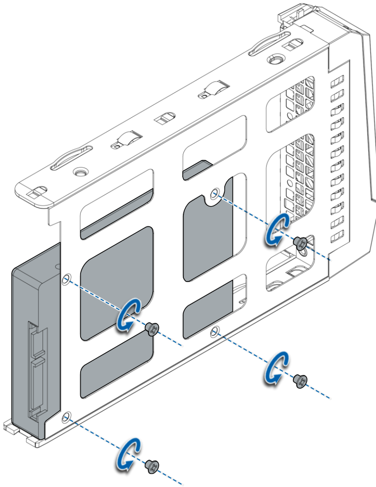
图 4-19 拆卸硬盘
