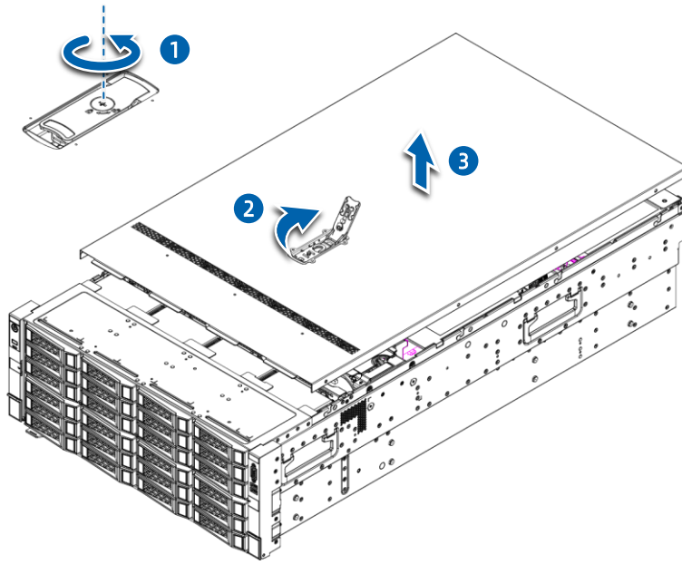
图 4-2 卸下机箱上盖
