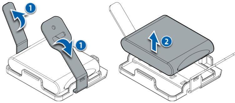
图 4-3 拆卸超级电容
