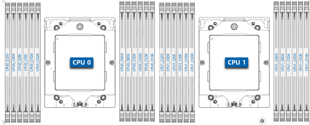
图 4-6 内存插槽布局
